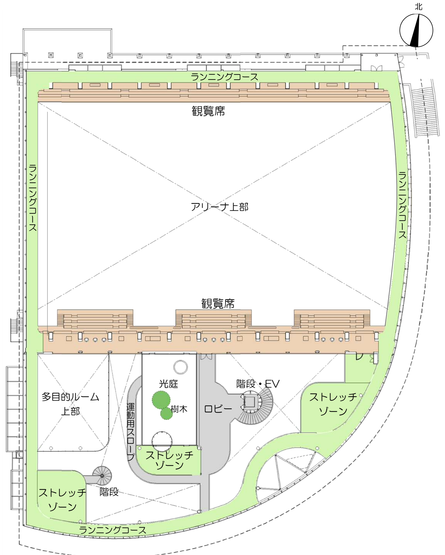
2階平面図
