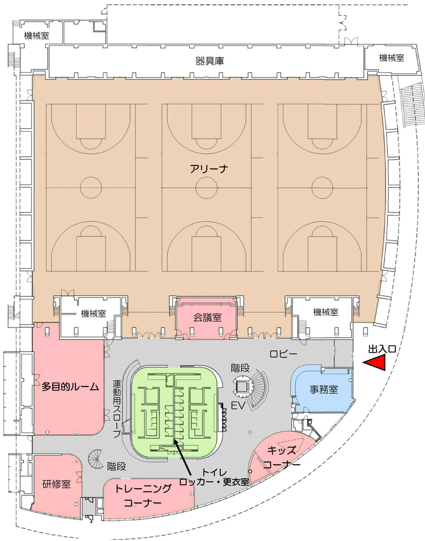
1階平面図
