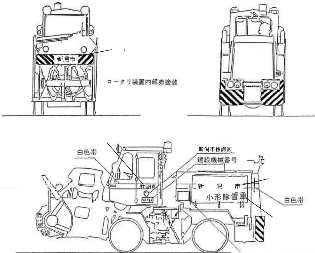
図4 除雪機械表示箇所図
