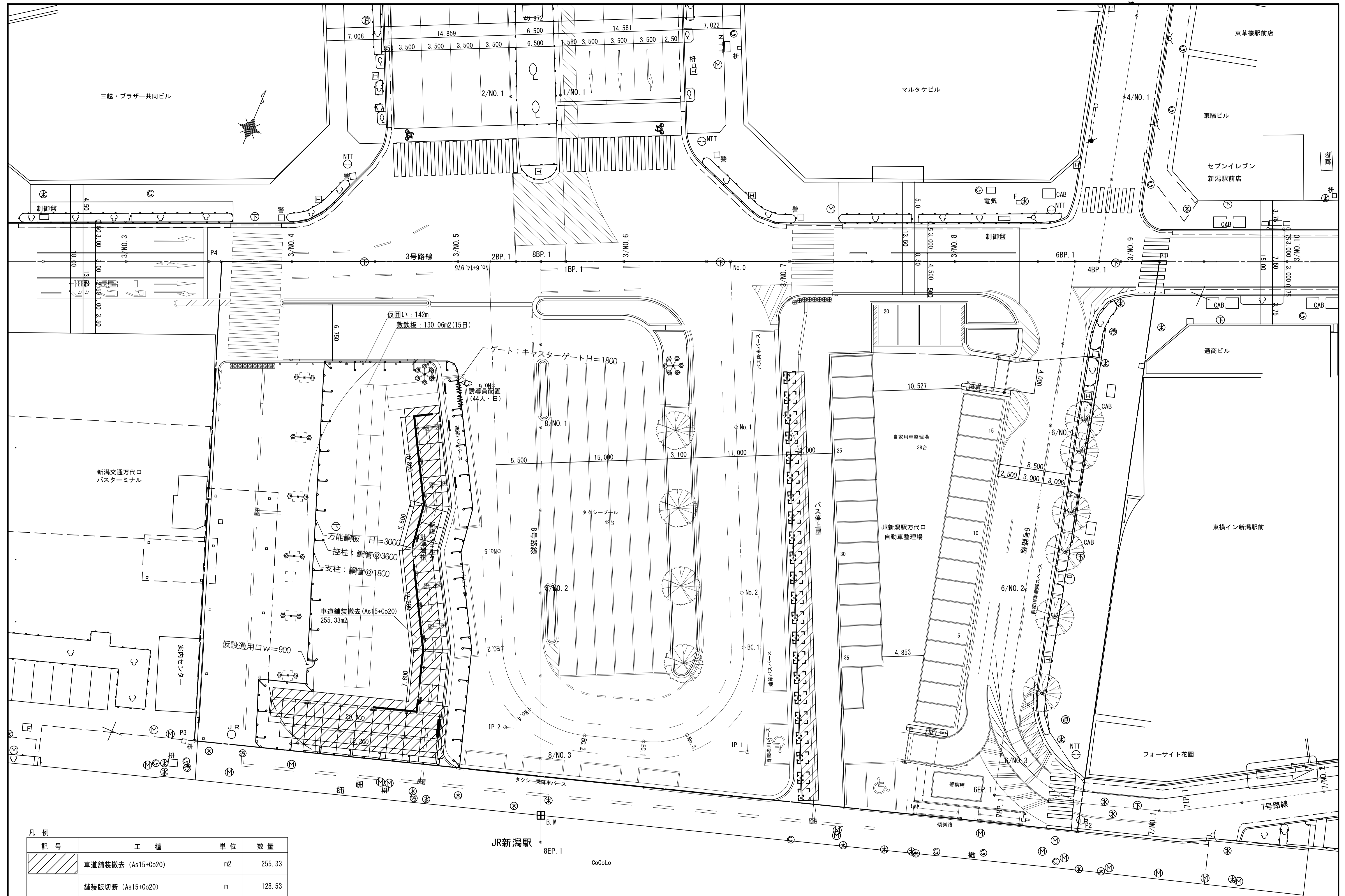
仮設計画図 S=1:200 (A3: S=1:400)
