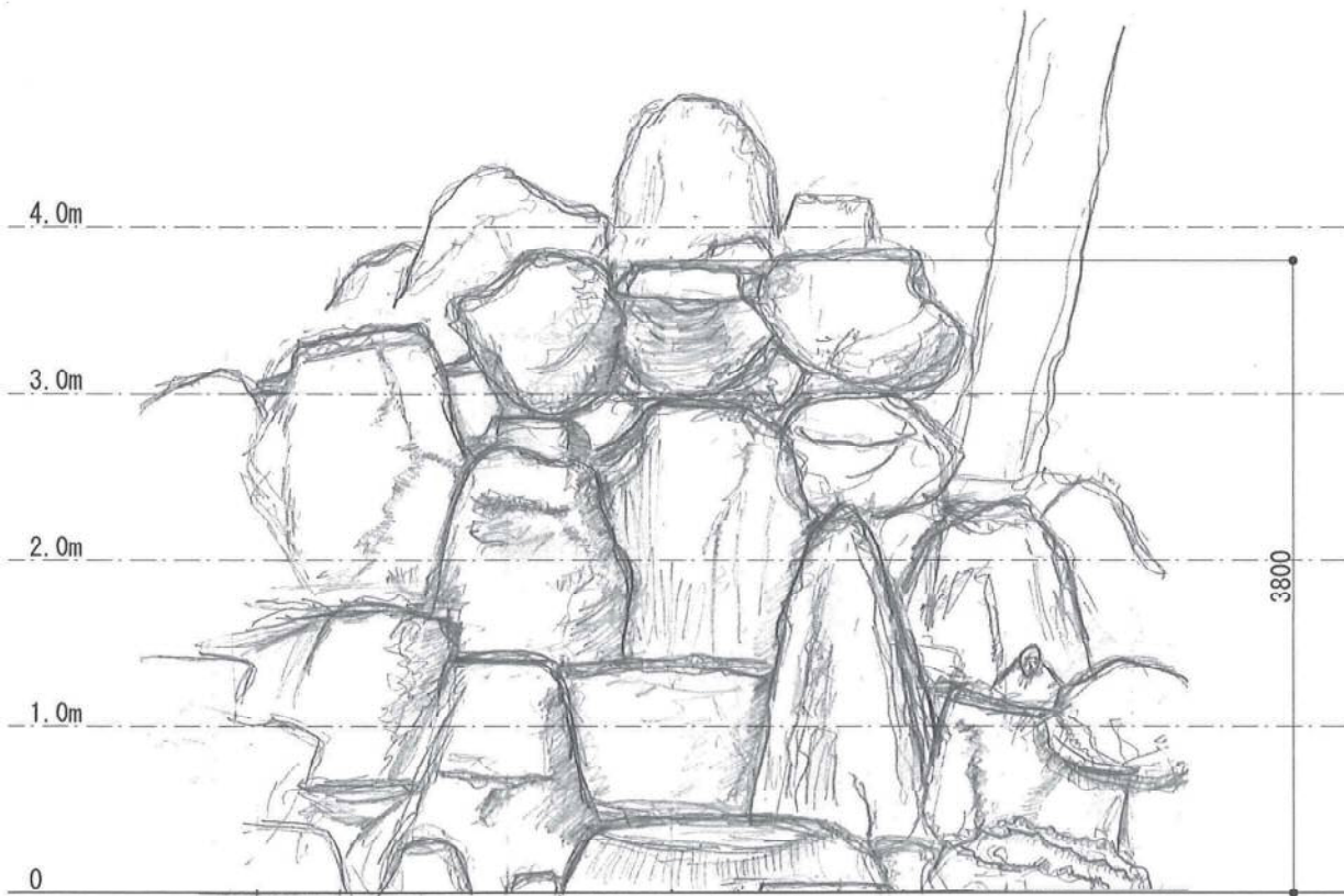
大瀧立面图 S=1/50
