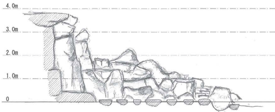
大瀧断面图 S=1/80
