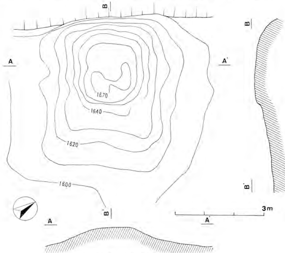
第3図 1号塚平面断面図
