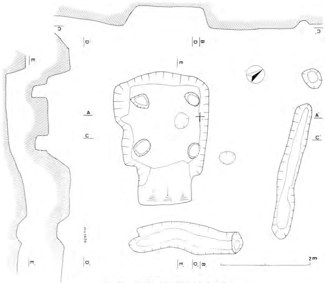
第5図 1号塚下層の竪穴式建物遺構
