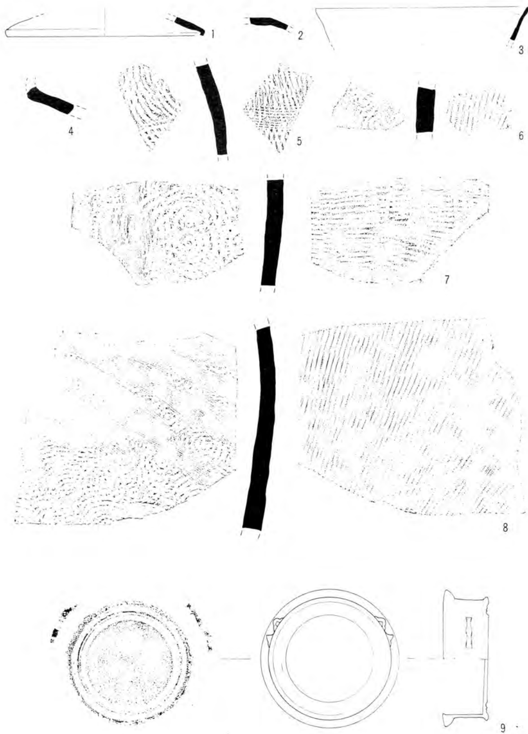
第7图 1号塚出土、土器(須惠器)鉦鼓 1/3
