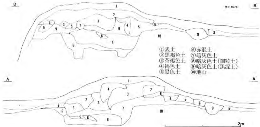
第4図 1号塚土層図
