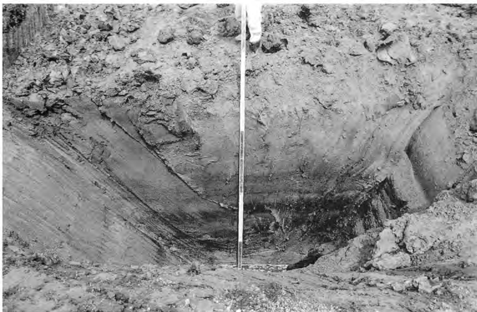
試掘坑 No. 1 土層
