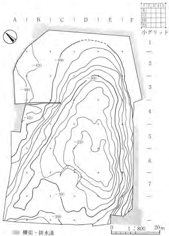
第3図 地形測量とグリッド設定図(1/800)
