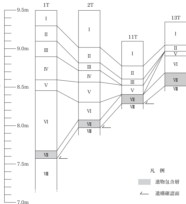
第3図 試掘坑土層柱状図(S=1/30)
