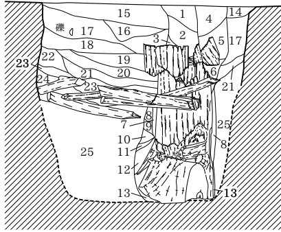
SX1378 (3J-8E3・4・8・9)
