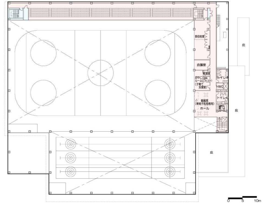
2階平面図
