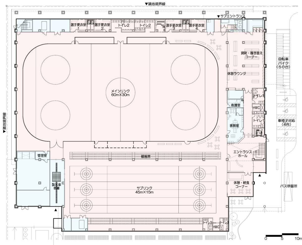
1階平面図
