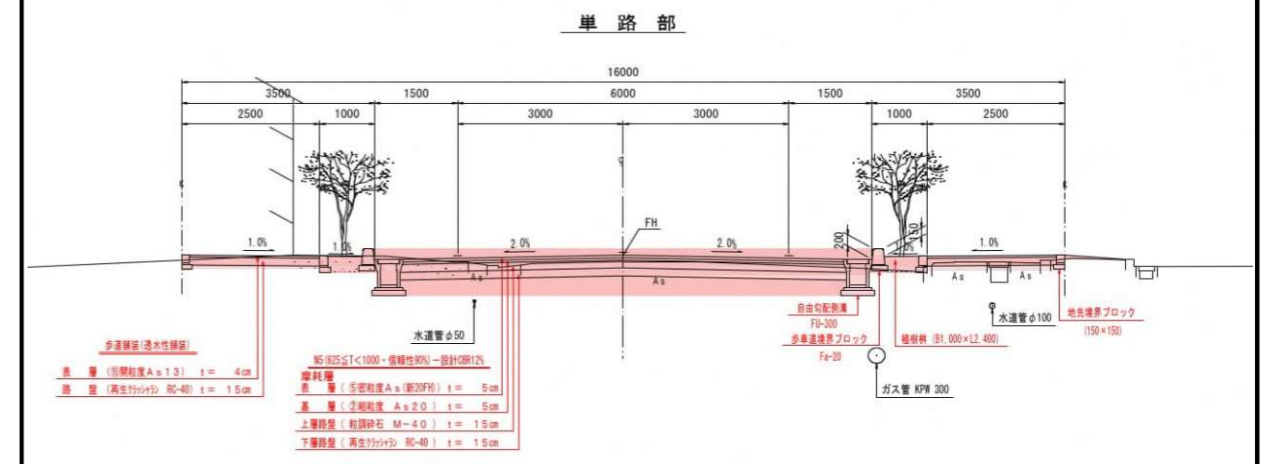
標準断面図
