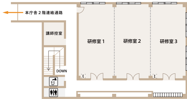
水道研修センター 2階平面図
