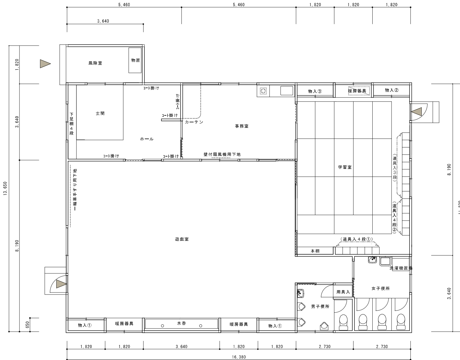
参考図 (1:100)
